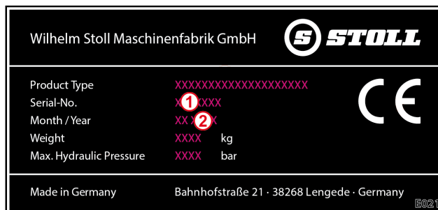
Abb. 1 / Fig. 1 Typenschild / Rating plate / Plaque signalétique
