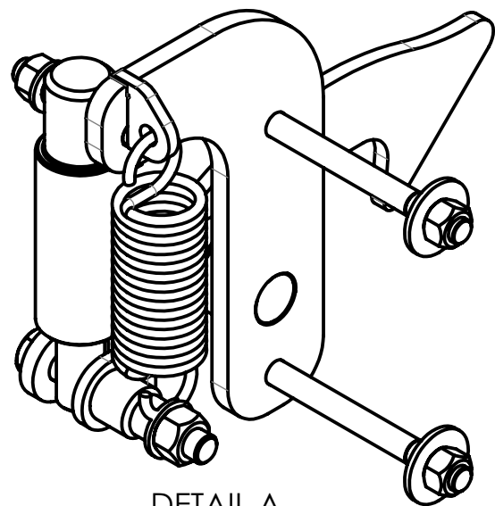
DETAIL A MAßSTAB 1 : 3
