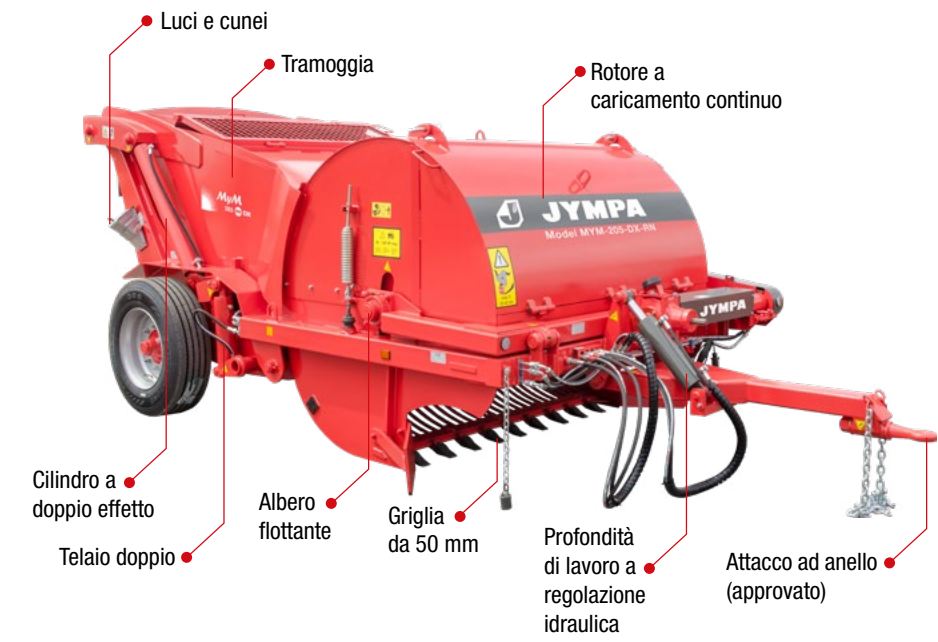
Modello MYM-205 DX
