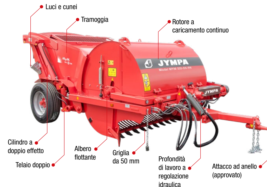
Modello MYM-205-AM-RN
