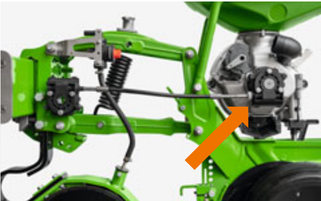
Con comando di singolarizzazione meccanico centrale SpeedShift
