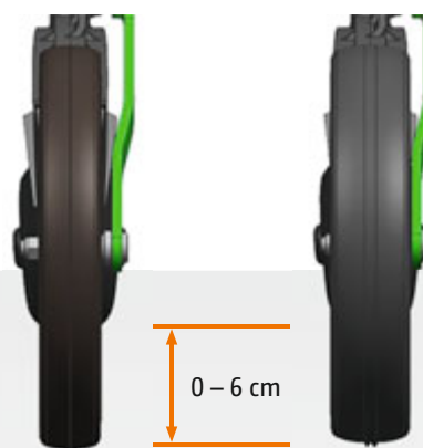
Profondità di lavoro dei rulli di guida in profondità Control 50 e Control 65
